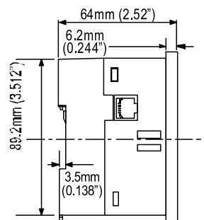
Рабочие размеры
