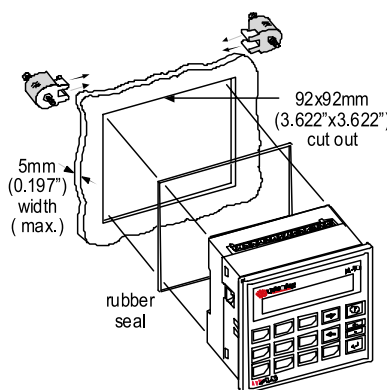
Установка в панель
