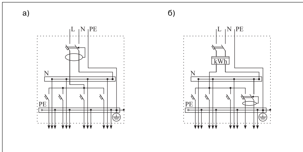
Схемы квартирных щитков (группового и учетно-группового), присоединенных к распределительным цепям, отходящим от: а) этажного учетно-распределительного щитка; б) этажного распределительного щитка
